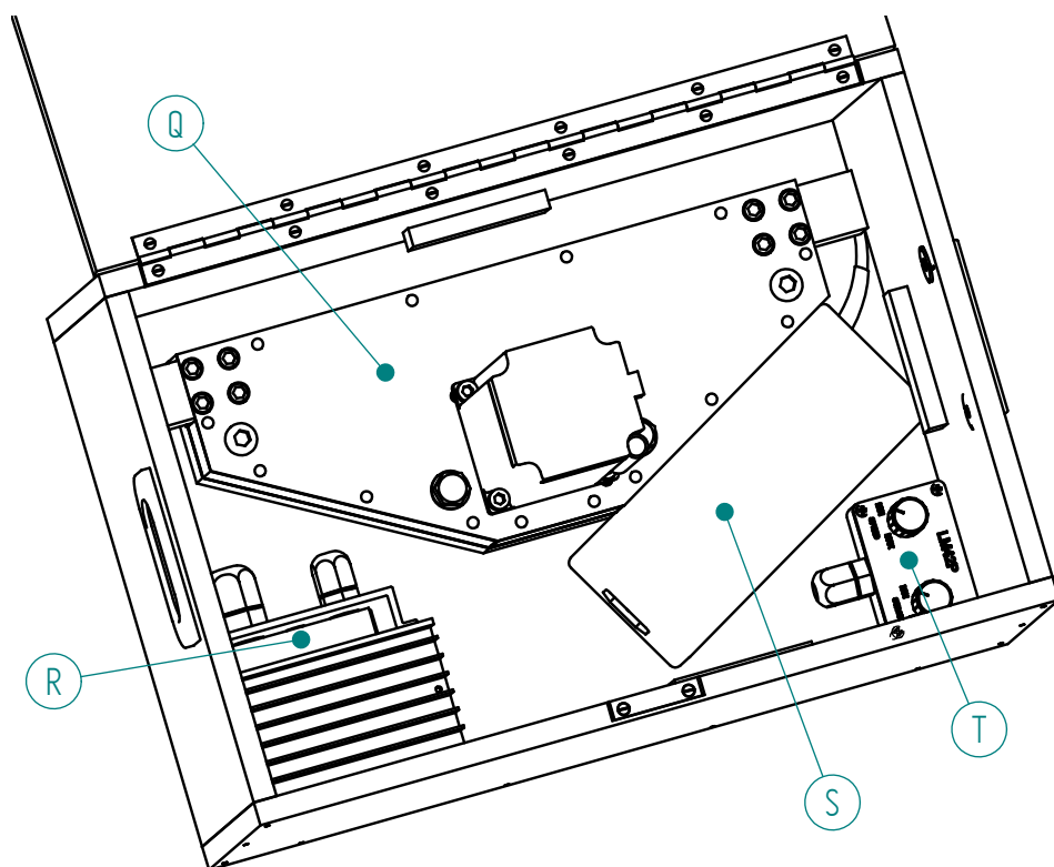
FIGURE 5 – Boîte de rangement sans le rack (fond de la boîte)
