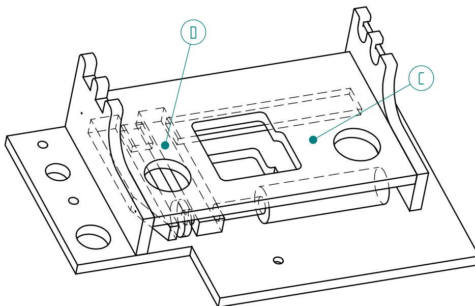
FIGURE 2 – Rack de rangement et emplacement du serre-joint
