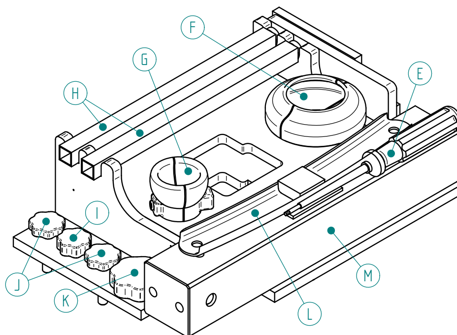
FIGURE 3 – Placement des éléments sur le rack
